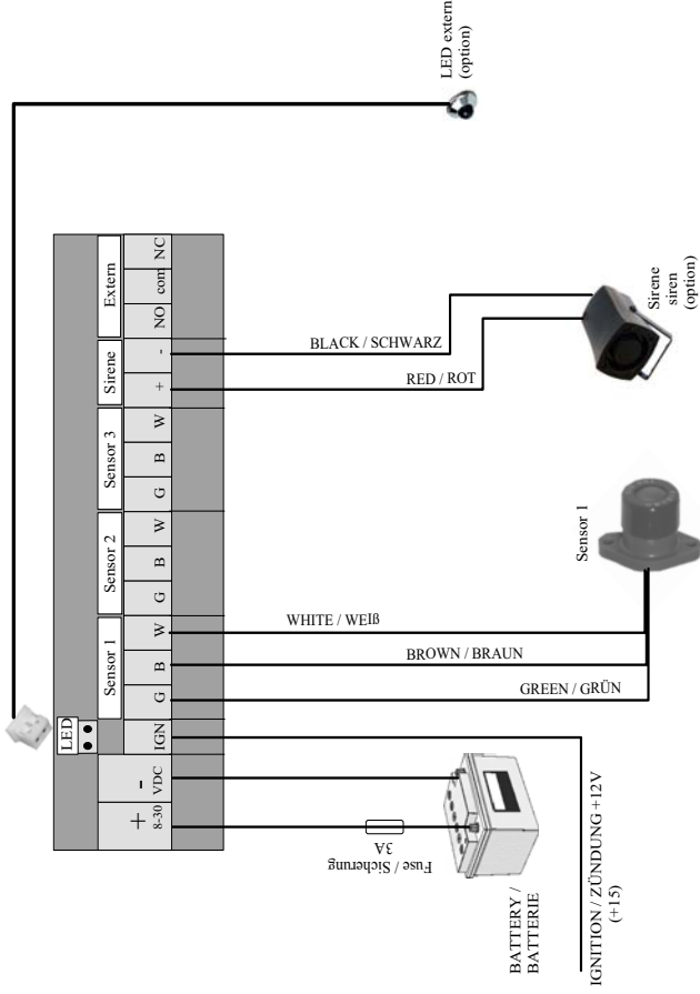
Abb.1 Anschlußplan:
